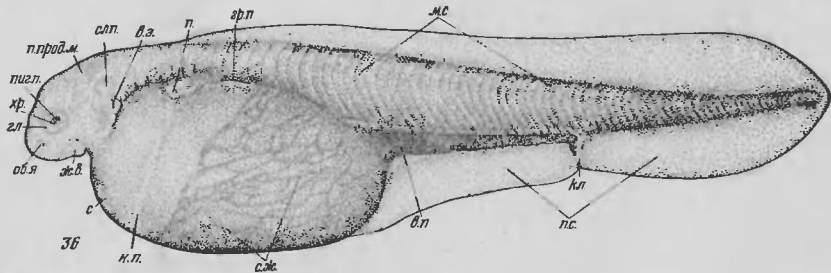
Рис. 47. Предличинка осетра после выхода из оболочек в период массового вылупления (ст. 36)
