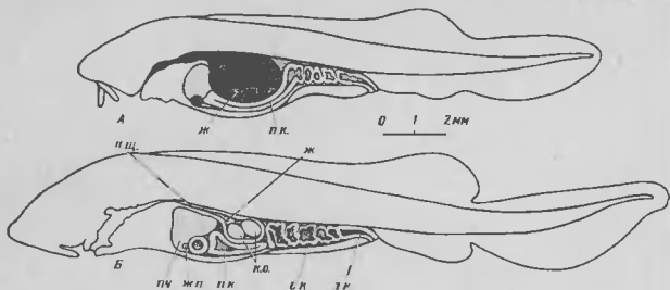
Рис. 59. Строение предличинки осетра, развивавшейся со стадий вылупления в присутствии кусочка латушной сетки (А) и одновозрастной контрольной личинки вскоре после перехода на активное питание (Б)
