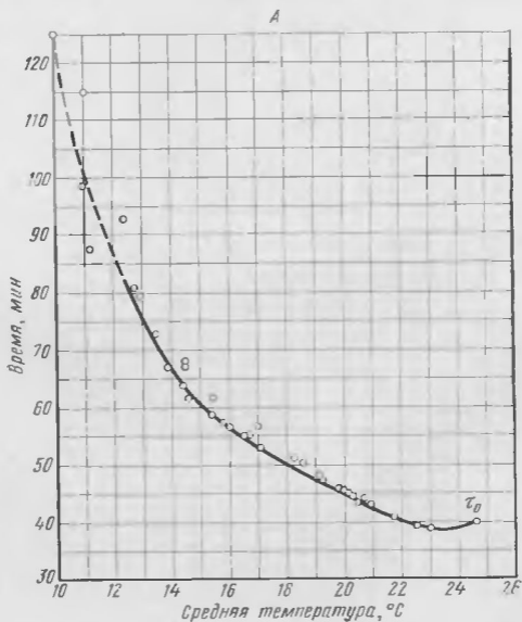
Рис. 28. Величина \tau_0 (продолжительность одного деления яйца в период синхронных делений дробления) у осетра (А), севрюги (Б) и белуги (В) при разных температурах (А, Б — Dettlaff, Dettlaff, 1961; В — Игумнова, 1975а)
