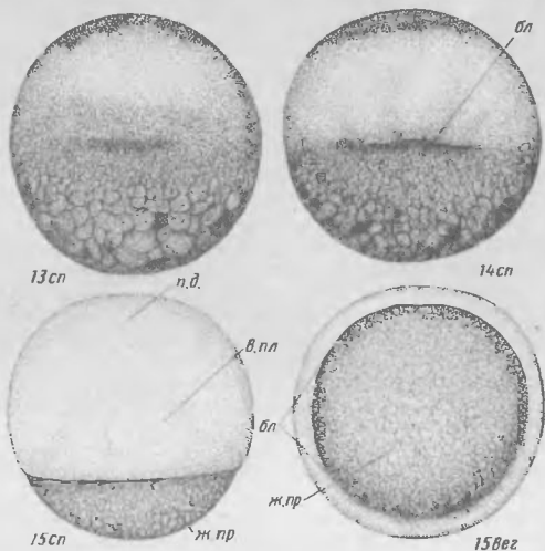
Рис. 31. Начало гастрюляции (ст. 13), ранняя гастрюла (ст. 14); средняя гастрюла (ст. 15)
