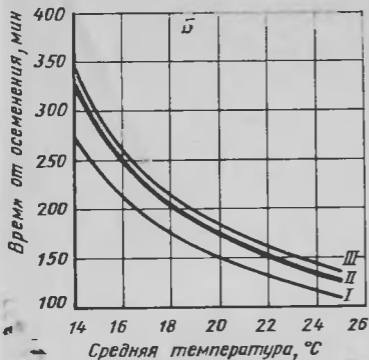
Рис. 64. Время взятия проб для определения процента оплодотворения яиц осетра (А), севрюги (Б) и белуги (В) в зависимости от температуры инкубации (А, Б — Деглаф, 1965а, В — Игумянова, 1975б)
