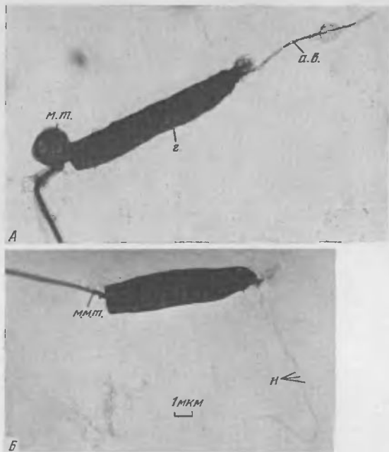
Рис. 19. Спермии черноморско-азовского осетра после осуществления акросомной реакции (электронно-микроскопические фотографии)
