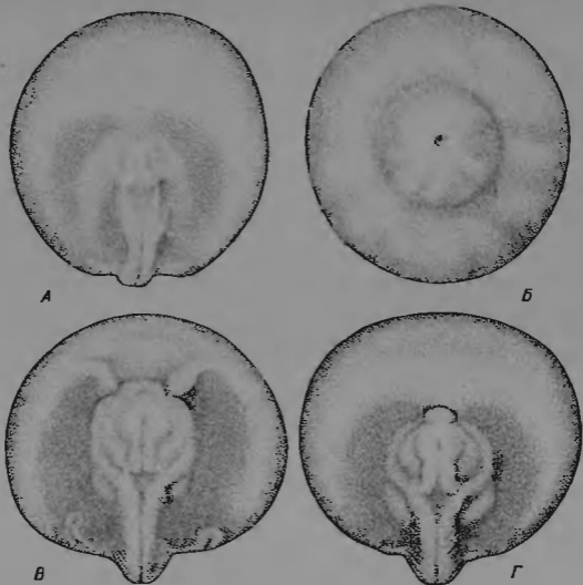
Рис. 40. Зародыши атипичного строения на стадиях 26 и 28 (Гинзбург, Деллаф, 1975)
