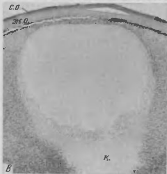
Рис. 5. Строение анимальной области ооцита осетра на последовательных стадиях созревания (Гинзбург, Деглаф, 1969). В скобках указано время от инъекции самке суспензии гипофизов до наступления указанных стадий в числе \tau_0 (см. ниже)
