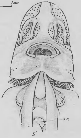
Рис. 53. Строение головы медличинки белуги (А, А') севрюги (В, В') на стадиях 3 (А, Б) и 45 (А', Б'); вид сверху
