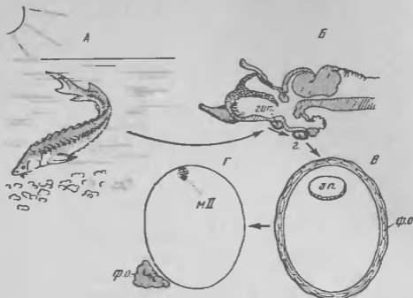
Рис. 1. Схема процессов, приводящих к созреванию ооцитов осетровых рыб (Гинзбург, Детлаф, 1969)
