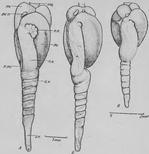
Рис. 56. Пищеварительная система предличинки осетра, развивавшихся со стадии вылупления в присутствии фенола (40 мг/л, Б) или кусочка латуинной сетки (В), и одновозрастная контрольная предличинка на стадии 45 (А) (А. Б.— Шмальгаузен, 1972)
