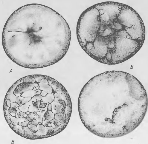
Рис. 30. Партеногенетическое дробление: начинающееся (А) и недалеко зашедшее (Б); предельная стадия дробления неоплодотворенных яиц (В) и отмирающее неоплодотворенное яйцо (Г) (Гиизбург, Детлаф, 1969)
