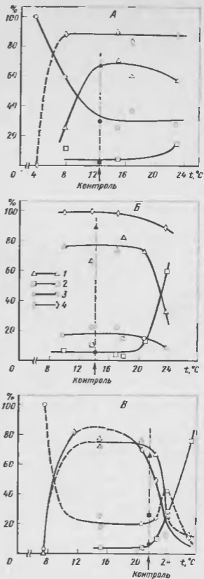
Рис. 7. Созревание ооцитов осетра в теле самки в растворе Рингера (Гинзбург, Детлаф, 1969)
