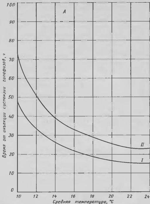
Рис. 62. Зависимость продолжительности созревания самок осетра (A), севрюги (B) и белуги (B) от температуры (B — Игумнова, 1974)
